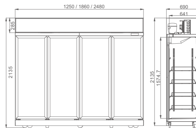
LG4-1160M2W / LG4-1860M3W / LG4-2360M4W
